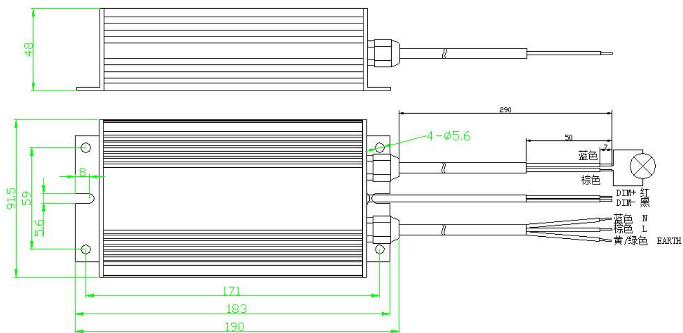
安装图与接线图
